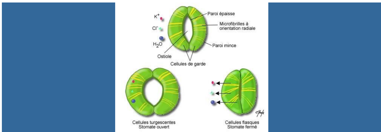
Figure n °9 : Schéma d'un stomate (A : Coupe longitudinale au niveau du parenchyme Chlorophyllien ; B : schéma général) montrant le stomate
