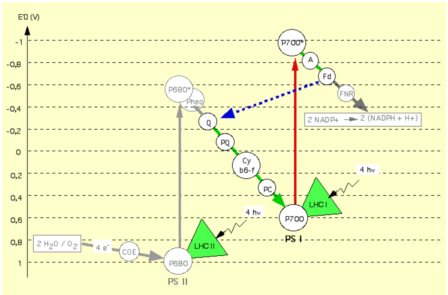
Figure n°18 : Transfert cyclique de électrons autour du PSI.
