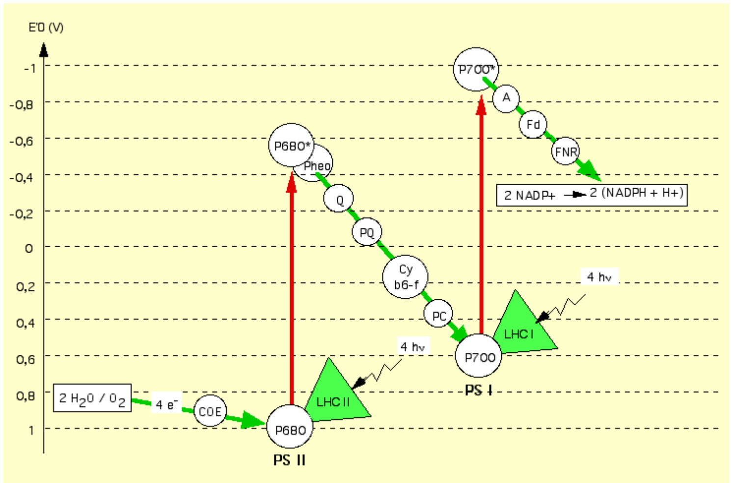
Figure n°17 : Schéma "en Z", transfert acyclique des électrons.
